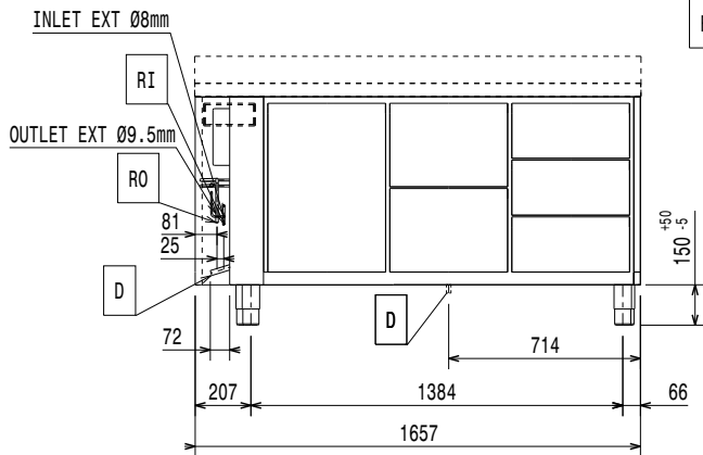
Zij aanzicht
